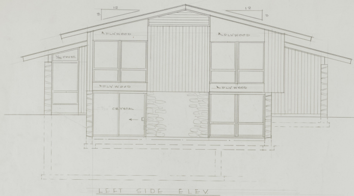
LEFT SIDE ELEV
