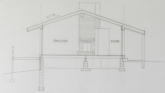
SECTION A-A 1/4"
