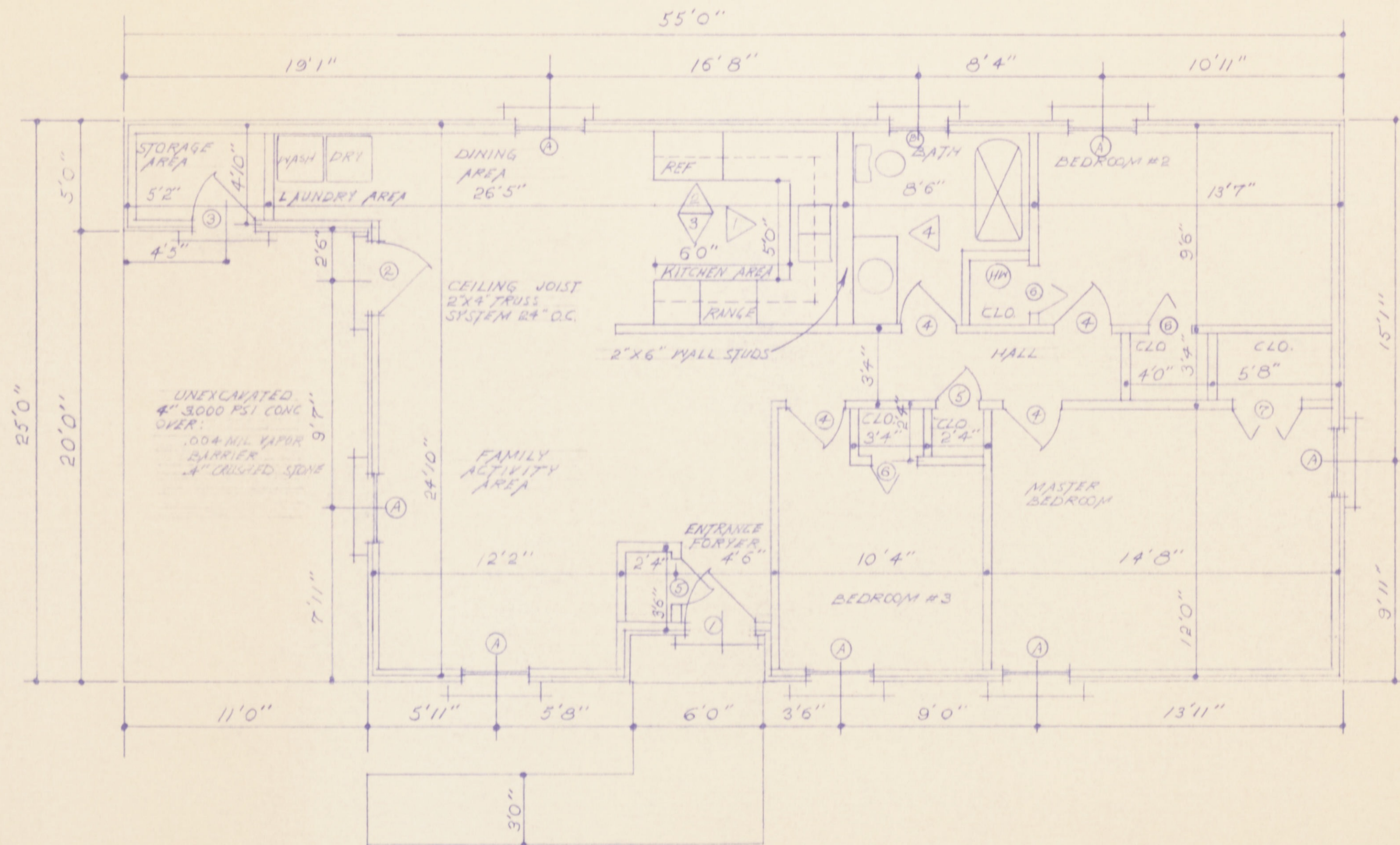
DOOR SCHEDULE
