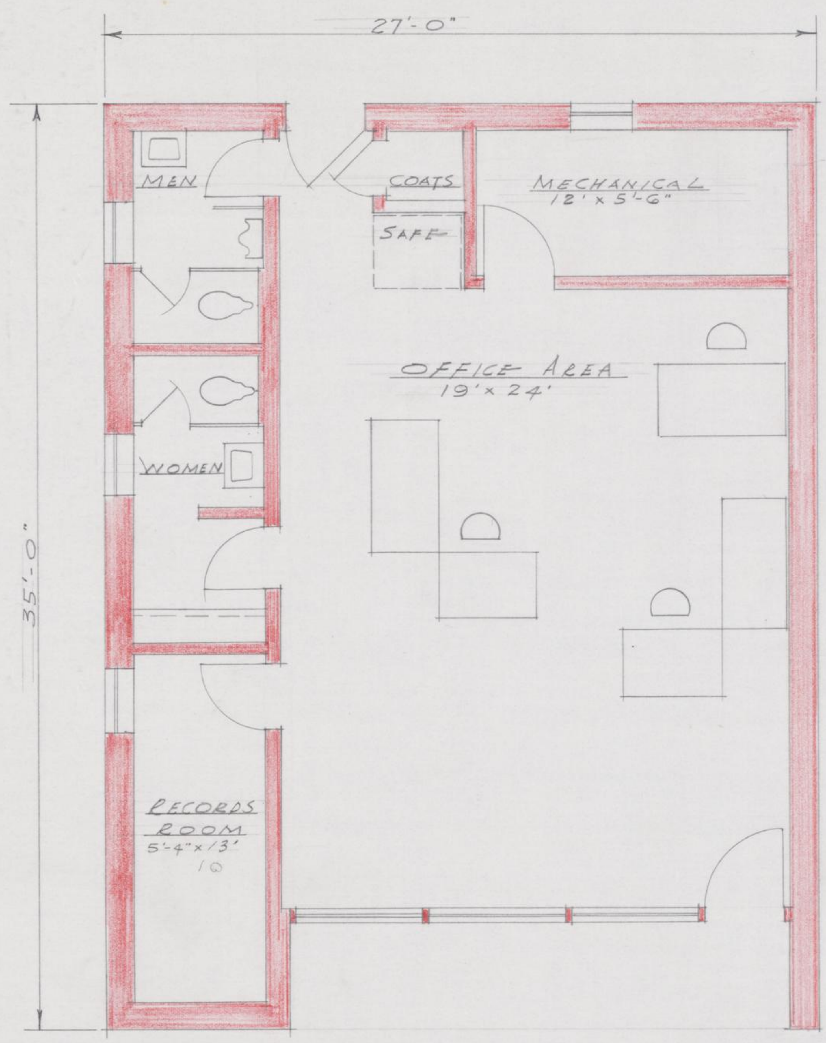
P L A N Sc. 1/4" = 1'-0"
